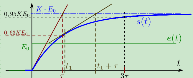
FIG. 1 – Réponse d'un 1 er ordre à un échelon
