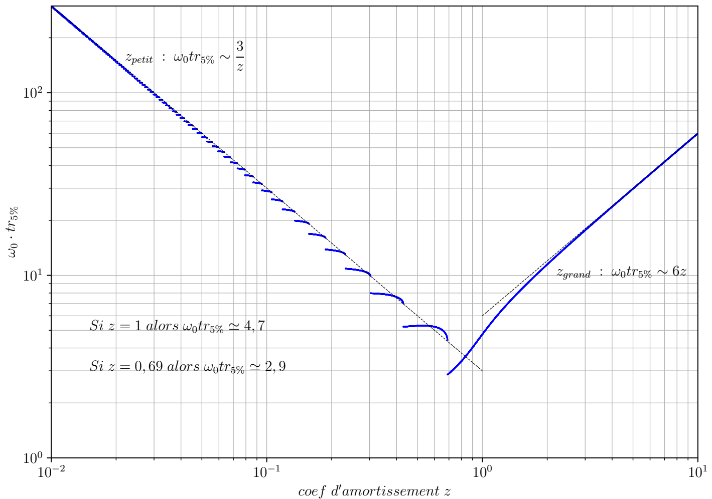
FIG. 4 – Temps de réponse à 5% d’un 2 d ordre
